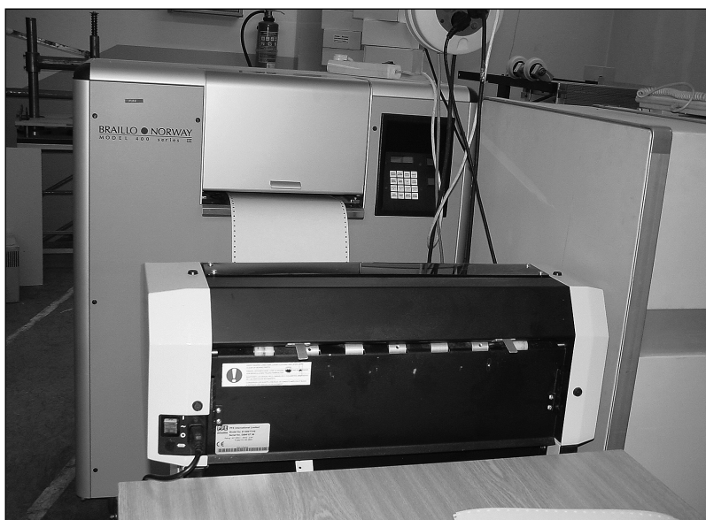
Norský elektronický sázecí stroj pro Braillovo písmo typu BRAILLO 400. Je ovládán z počítače, ve kterém je text vysázen digitálně. Nepoužívá proto matic ani lisu. Tiskne přímo na papír, který se odvíjí z role.
