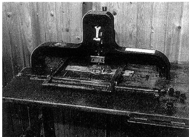
Sázeční stroj pro tisk Braillovým písmem
