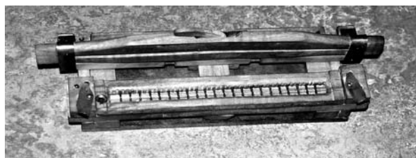
Pomůcka pro psaní Braillovým písmem
