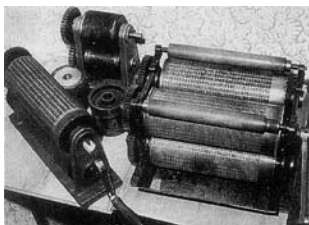
Rozmnožovací rotačkové zařízení pro tisk Braillovým písmem
