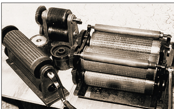
Ladislav Korunka, ruční rotačka pro Braillovo písmo
